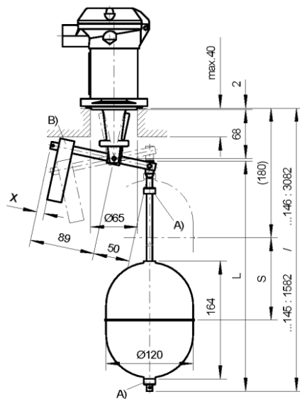
Dibujo técnico módulo de flotador -145 / -146
