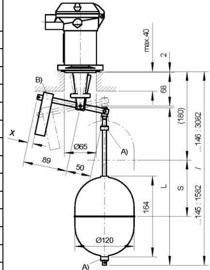
Massbild Schwimmermodul -145 / -146
