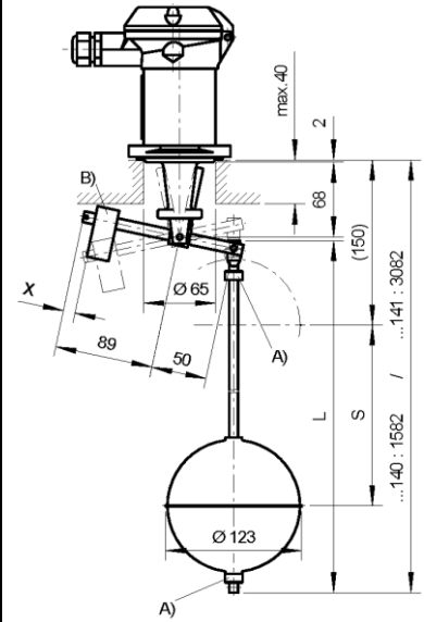
Massbild Schwimmermodul -140 / -141
