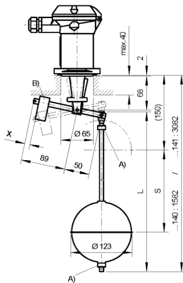
Dibujo técnico módulo de flotador -140 / -141
