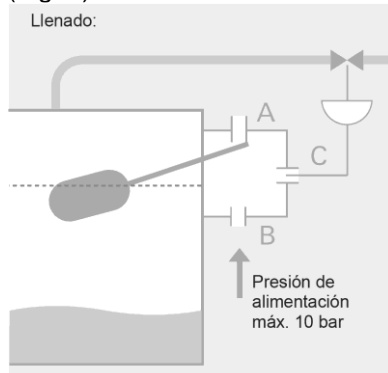
(Fig. 1) Llenar
