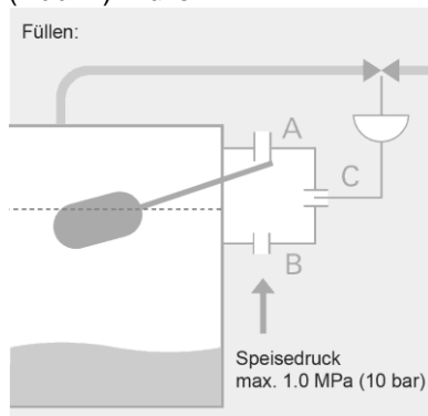
(Abb. 1) Füllen
