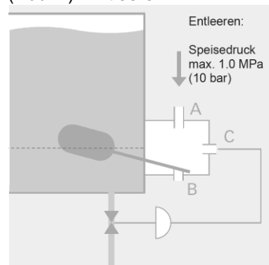
(Abb. 2) Entleeren
