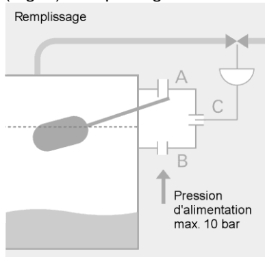
(Fig. 1) Remplissage
